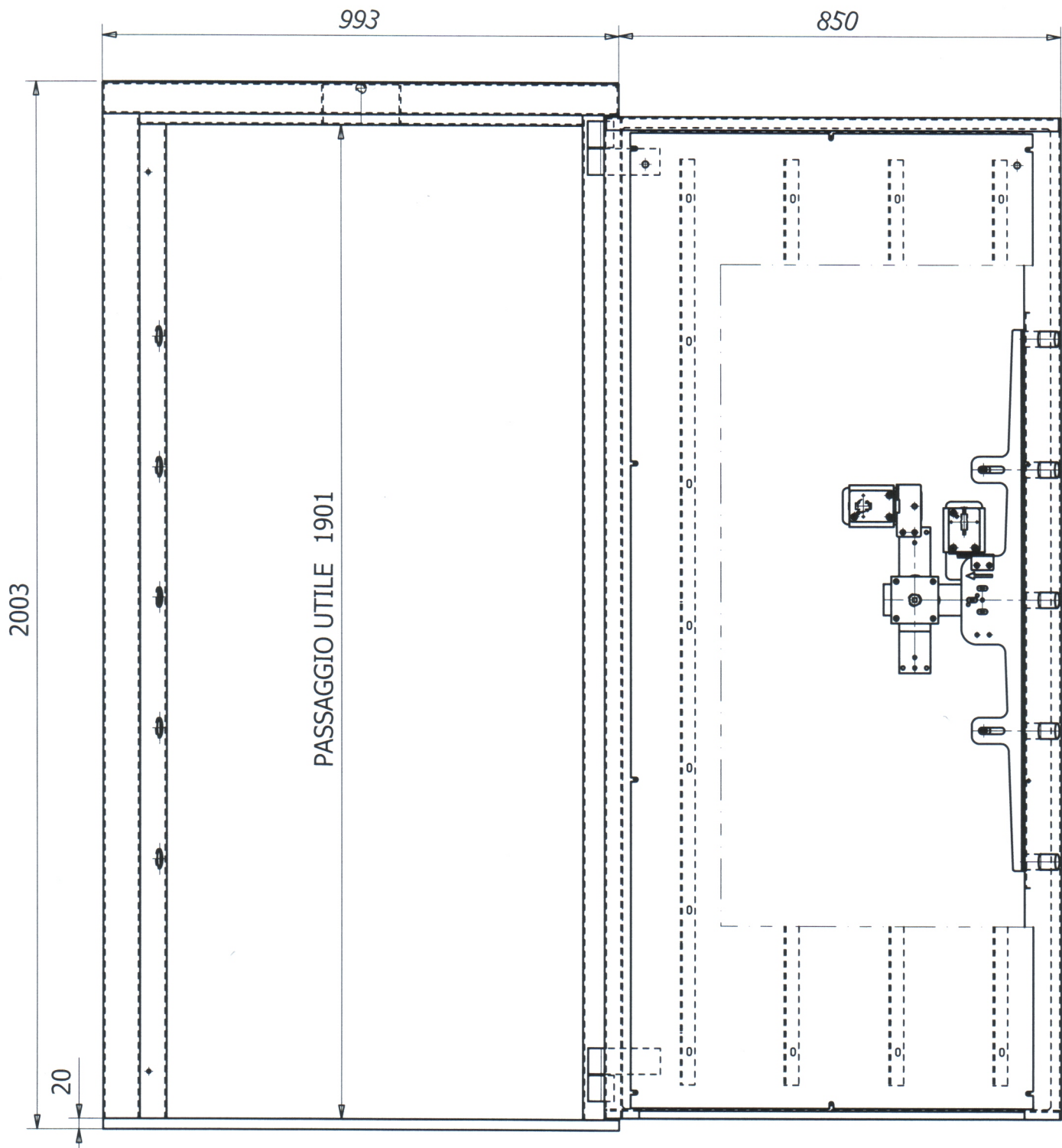
PORTA CORAZZATA PC 1900 SCHEMA GENERALE
