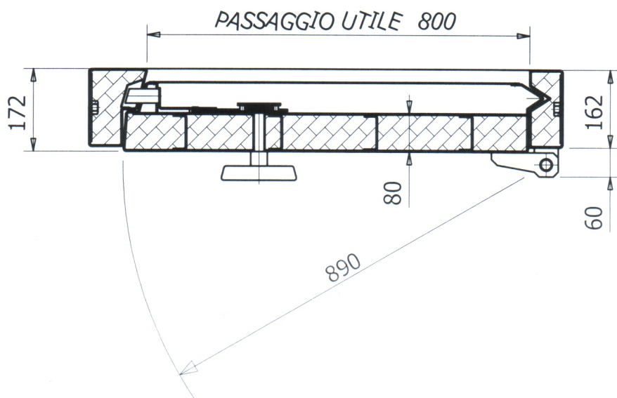
PORTA CORAZZATA PC 1900 SCHEMA GENERALE
